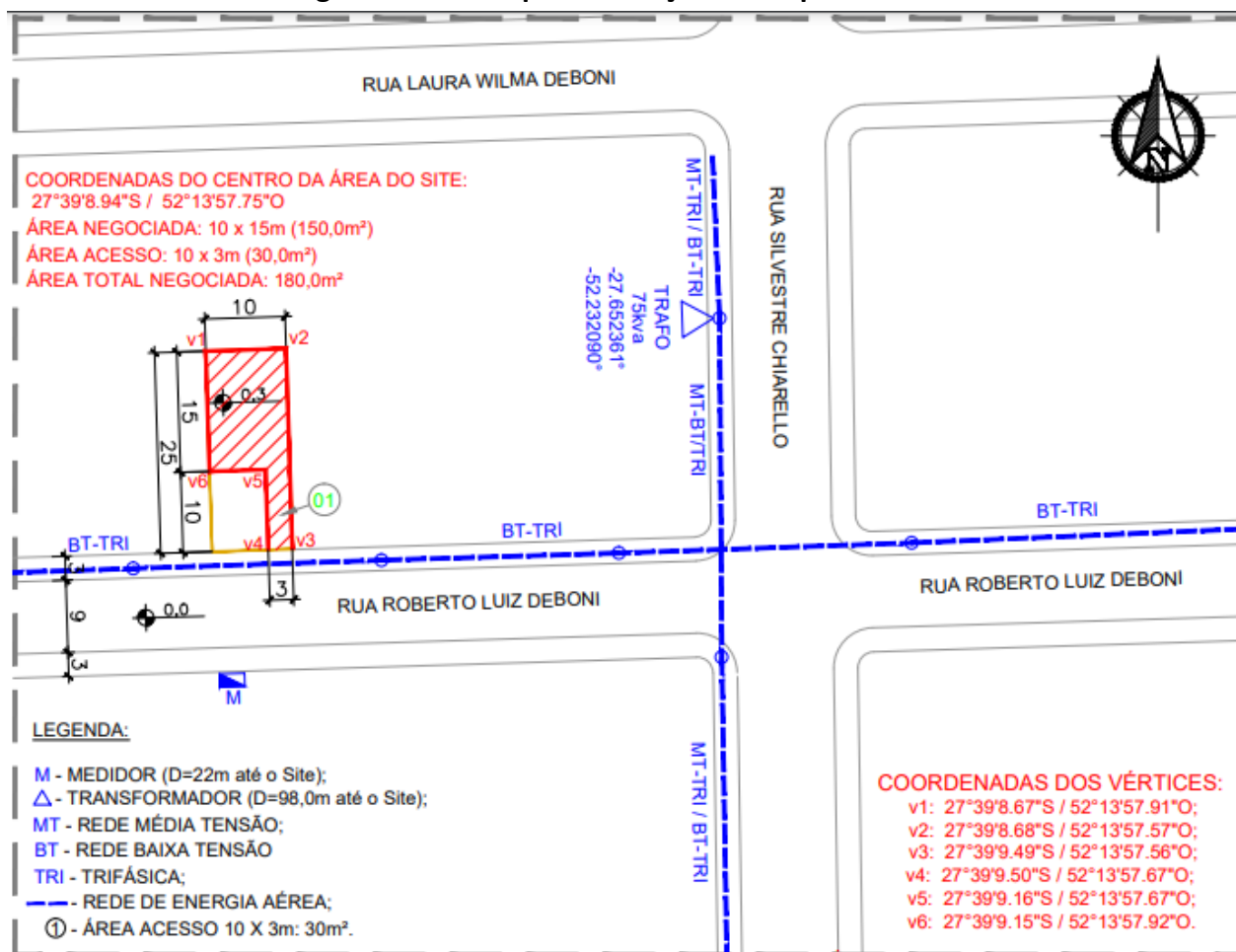
Figura 02.1 – Croqui de situação do empreendimento
